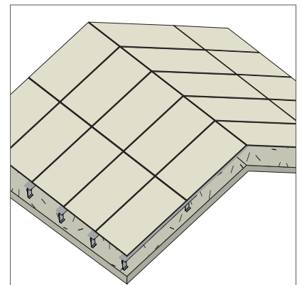
Cobertura ventilada
